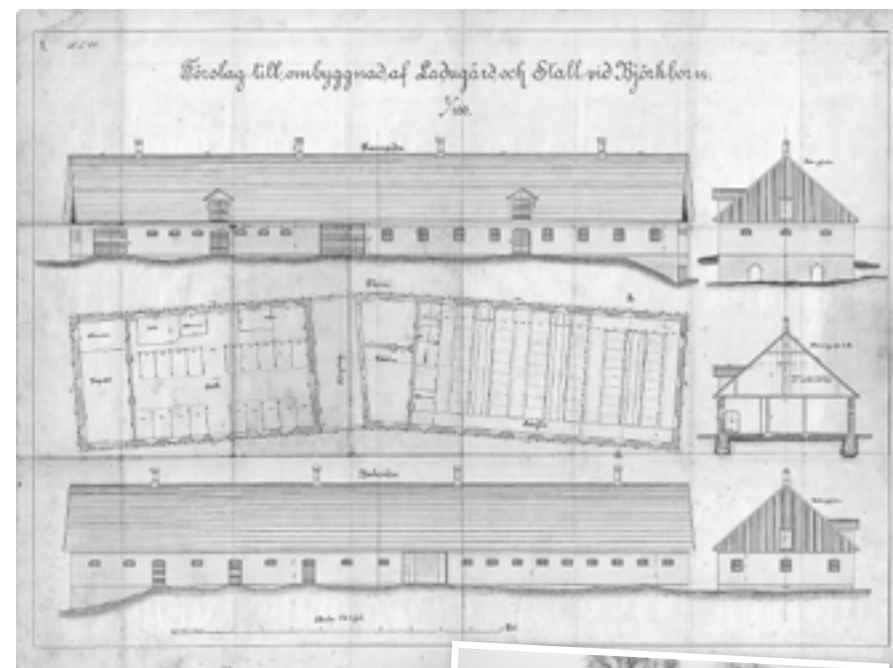
En gammal ritning från 1800-talets slut på "Förslag av ombyggnad af Ladugård och Stall vid Björkborn". Foto Hans Johansson
